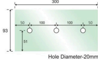
DFP-300 Fin Plate 300mm
