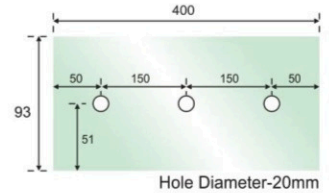
DFP-400 Fin Plate 400mm
