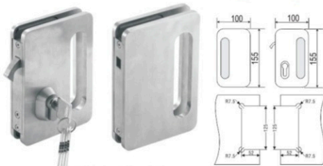
DSDL-13A+13B Sliding Door Lock+Strike Box
