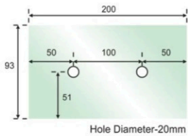
DFP-200 Fin Plate 200mm
