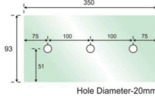
DFP-350 Fin Plate 350mm
