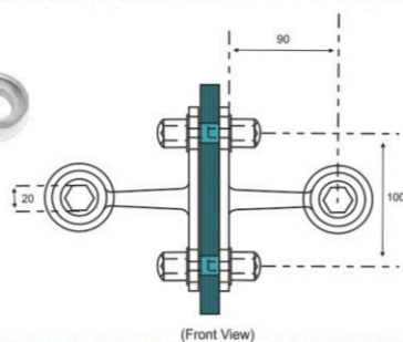
DSP-A2 2 Way Spider 180° with Fin
